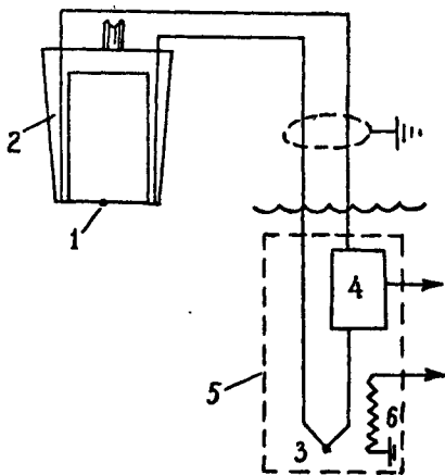
Рис. 3.12. Конструкция и электрическая схема датчика температуры
