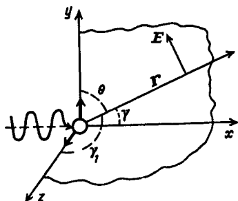
Рис. 2.13. Излучение двух взаимно ортогональных линейных гармонических осцилляторов
