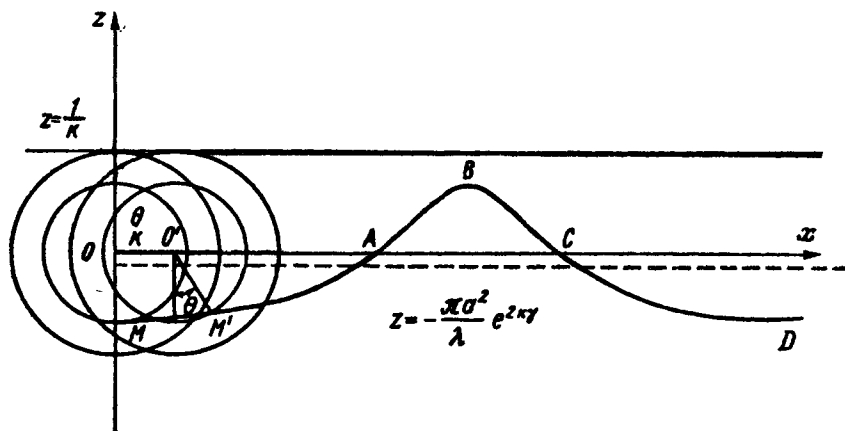
Рис. 2.8. Волна трохоидалного профиля: сплошная прямая линия — положение невозмущенного уровня воды, пунктир — геометрическое место центров круговых орбит поверхностных частиц воды
