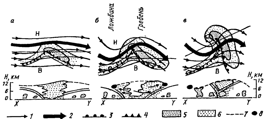
Рис. 6.3. Стадии развития (а, б) и окклюдирования (в) циклона. Верхний ряд — эволюция циклона на синоптической карте. Нижний ряд — вертикальные разрезы циклона по линиям xу , указанным на верхних рисунках тонкими прямыми линиями. 1 — линии верхних течений, 2 — струйное течение, 3 — теплый фронт, 4 — холодный фронт, 5 — области осадков, 6 — облачность без осадков, 7 — тропопауза, 8 — сечение струйного течения; Н — низкое давление, В — высокое давление
