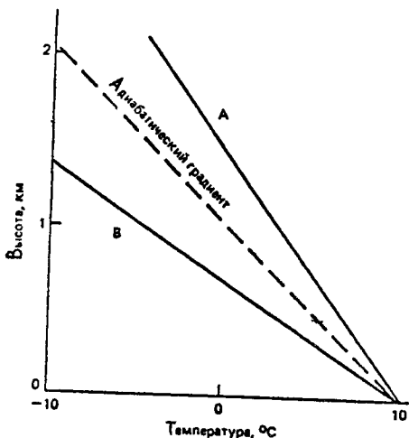
Рис. 1.8. Графики, отражающие условия устойчивости (A) и неустойчивости (B) в атмосфере
