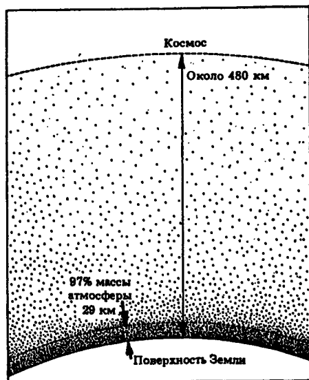
Рис. 1.2. Вертикальное распределение массы атмосферы
