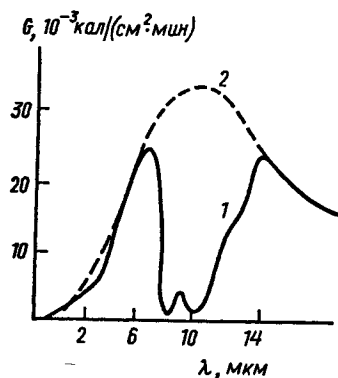
Рис. 3.3. Спектры излучения атмосферы (1) и подстилающей поверхности (2) при температуре, близкой к нормальной ( \sim 300 \text{ К} )
