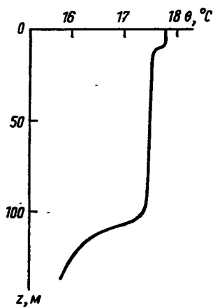
Рис. 3.6. Характерный профиль температуры в деятельном слое океана
