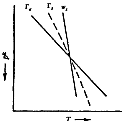
Рис. 1.12. Псевдоадиабатическая диаграмма: \Gamma_a — адиабатическая кривая, \Gamma_s — псевдоадиабатическая кривая и w_s — кривая постоянного отношения смеси при насыщении
