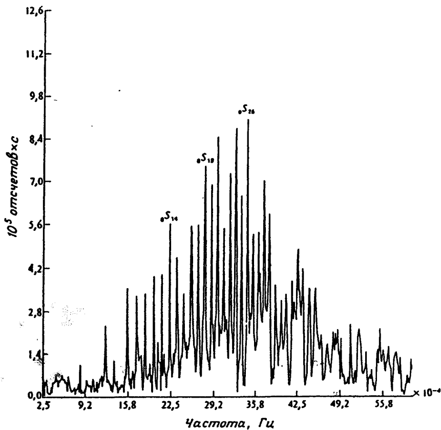
Рис. 2.12. Запись собственных колебаний Земли на сейсмограмме землетрясения в Индонезии 19 августа 1977 г. (магнитуда 7.9), частотный спектр (б), рассчитанный по сейсмограмме (а) (по Болту, 1984)
