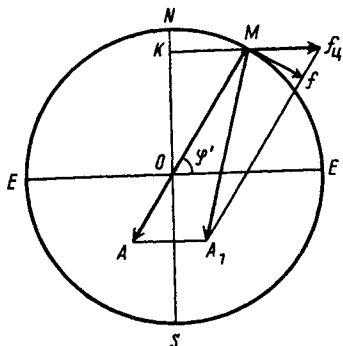
Рис. 1.1. Модель круглой вращающейся Земли. MA — сила тяготения, f_{ц} — центробежная сила, f — горизонтальная проекция f_{ц} , направленная к экватору
