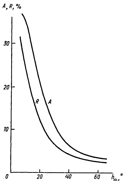
Рис. 2.19. Изменение с высотой Солнца h_{\odot} альбеда океана ( A ). Для сравнения приведена кривая изменения коэффициента отражения R
