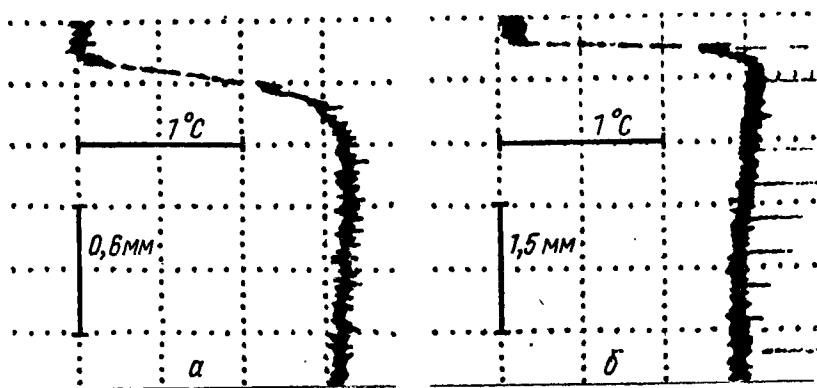
Рис. 3.20. Профили температуры в холодной пленке: a — при шквальном ветре со скоростью 20 м/с; b — при обдуве поверхности моря струей воздуха со скоростью 40 м/с
