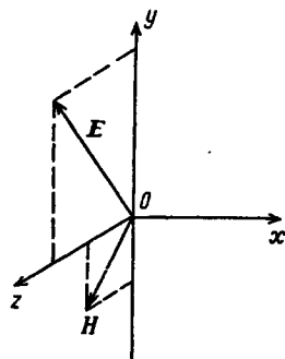
Рис. 2.9. Распространение плоской электромагнитной волны в положительном направлении x с произвольной линейной поляризацией вектора напряженности электрического поля E
