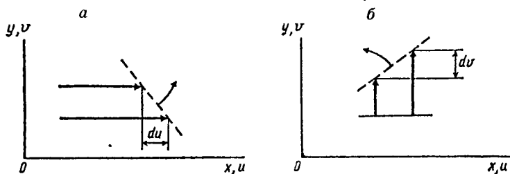
Рис. 6.2. Составляющие вихря: а — \frac{du}{dy} < 0 , б — \frac{dv}{dx} > 0
