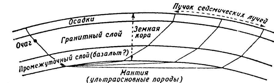
Рис. 2.6. Ход сейсмического луча от близкого землетрясения в слоистой земной коре
