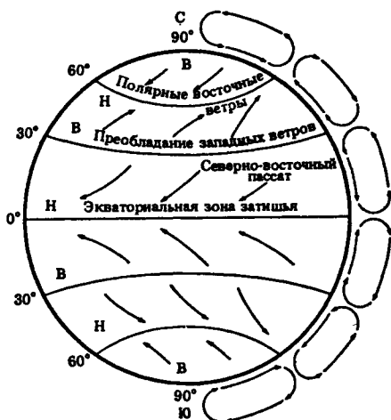
Рис. 3.31. Схема распределения поясов высокого (В) и низкого (Н) давления и ветров на земном шаре
