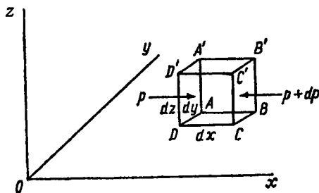
Рис. 5.1. Расчет силы, обусловленной градиентом давления
