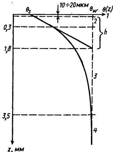
Рис. 3.19. Модель холодной пленки
