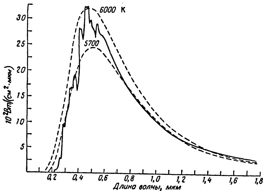
Рис. 2.3. Наблюдаемый солнечный спектр (сплошная линия) и спектральная интенсивность излучения черного тела при температуре 6000 и 5700 К (пунктирные линии)
