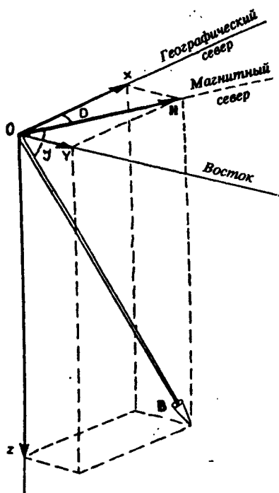
Рис. 4.1. Схема определения геомагнитной индукции B в некоторой точке O с географическими координатами (\varphi, \lambda) . Проекции H, X, Y, Z и углы D (магнитное склонение) и J (магнитное наклонение) — элементы геомагнитного поля
