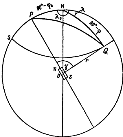
Рис. 4.6. Схема земного магнитного диполя (по Б.М. Яновскому, 1978)
