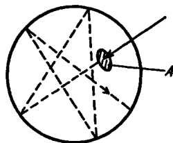
Рис. 2.2. Модель черного тела
