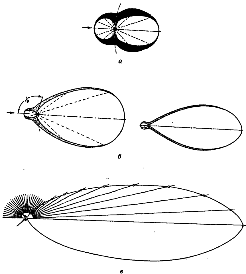
Рис. 3.1. Индикатрисы рассеяния света для частиц различной крупности: а — размер частицы сравним с длиной волны падающего излучения; б — более крупные частицы; в — предельно большая частица (по В.В. Шулейкину, 1968)
