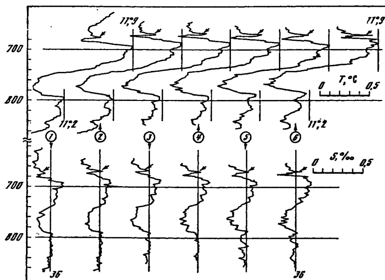
Рис. 1.4. Вертикальные профили температуры и солености по данным многократного зондирования с дрейфующего судна с интервалом в 6 мин в слое красноморских вод, распространяющихся в толще вод Аравийского моря (Океанология. Физика моря, 1978)
